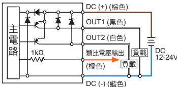
EP43□ - 030 - □ 2PNP + Analog 輸出 (1 ~ 5 V)
