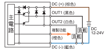
EP43□ - 04 - □ 2PNP + 複製功能
