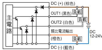
EP43□ - 031 - □ 2PNP + Analog 輸出 (4 ~ 20 mA)
